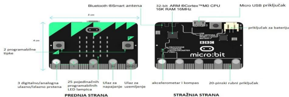
Slika 1: Shematski prikaz Micro:bita
